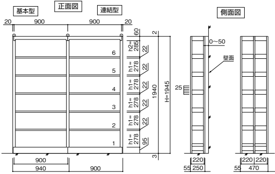
HM22 棚奥行D220タイプ
