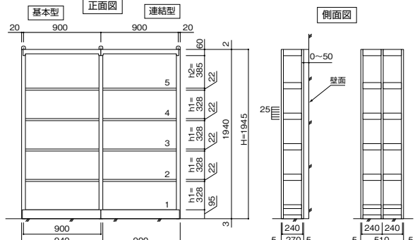
HM24 棚奥行D240タイプ
