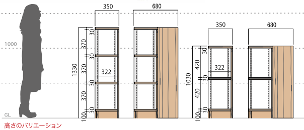
高さのバリエーション
