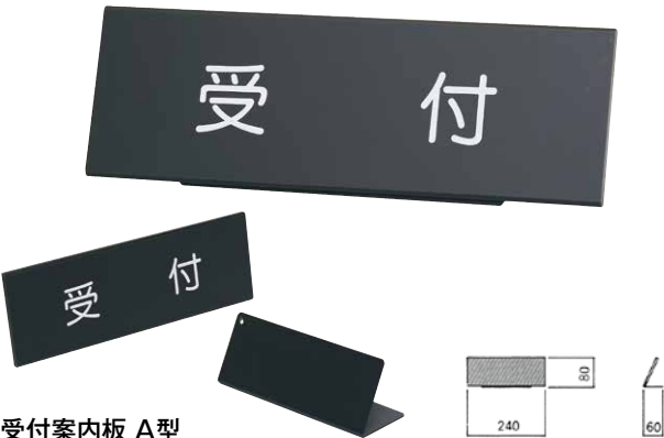
受付案内板 A型 4332 W240 × D60 × H80 ¥15,400+税 画面サイズ: W240×H80 表示基板: アクリル 表示基板色: アイボリー、ダークグレー フレーム: スチール (t=1.2) 焼付塗装 着脱方式: スライド 文字選択: 受付、貸出、返却
