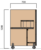
AVブースA型 2人用 7008 W1200 × D700 × H1200 ¥524,400+税
