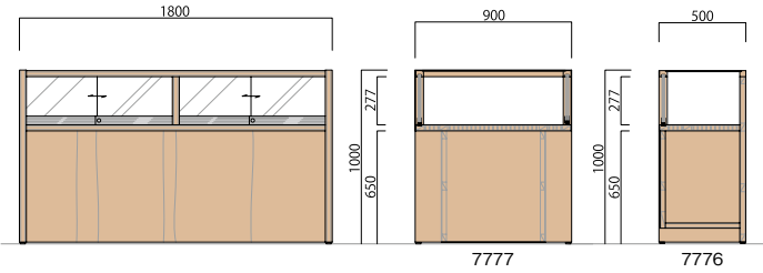
木製展示ケースN型 7776 片面 W1800 × D500 × H1000 ¥502,000+税 7777 両面 W1800 × D900 × H1000 ¥795,000+税
