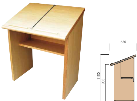
新聞閲覧台 A型 7370 1連 W900 × D650 × H1150 ¥255,200+税 7371 2連 W1800 × D650 × H1150 ¥380,000+税
