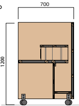
AVブースA型 1人用 7009 W900 × D700 × H1200 ¥475,000+税
