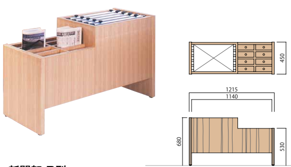
新聞架 B型 7348 W1215 × D450 × H680 ¥262,900+税 サスペンダー専用、5本掛及び新聞差し8個付です。(サスペンダーは別売です)
