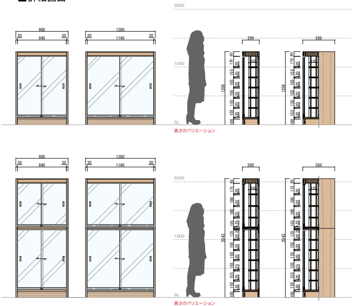
■詳細図面
