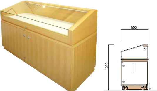
木製展示ケースM型 7779 W1600 × D600 × H1000 ¥760,000+税 材質:IR材 照明付、収納棚付、背面開閉式
