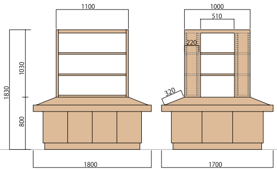
新刊展示架 C型 7685 W1800 × D1700 × H1830 ¥1,200,000+税 材質:IR材 棚板可動調節:N金具、棚受柱式(12.5mmピッチ)
