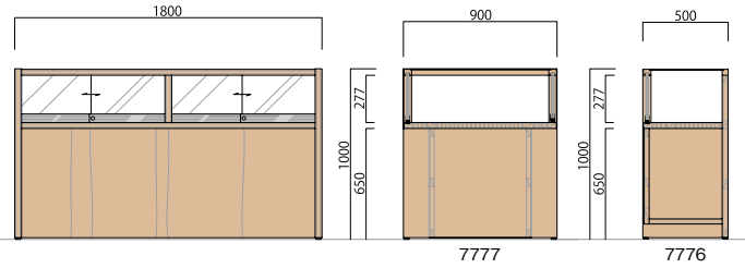
木製展示ケースN型 7776 片面 W1800 × D500 × H1000 ¥502,000+税 7777 両面 W1800 × D900 × H1000 ¥795,000+税 材質:IR材
