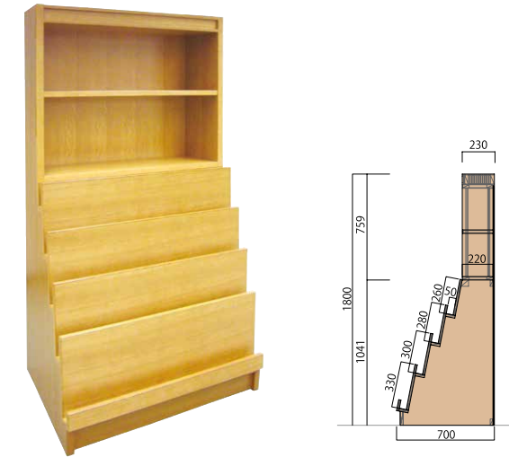
新刊展示架 A型 7630 W900 × D700 × H1800 ¥474,000+税 材質:IR材 棚板可動調節:N金具、棚受柱式(12.5mmピッチ)
