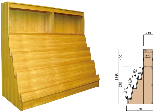
新刊展示架 B型 7635 W1600 × D570 × H1345 ¥622,500+税 材質:IR材
